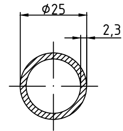
Querschnitt M2:1
