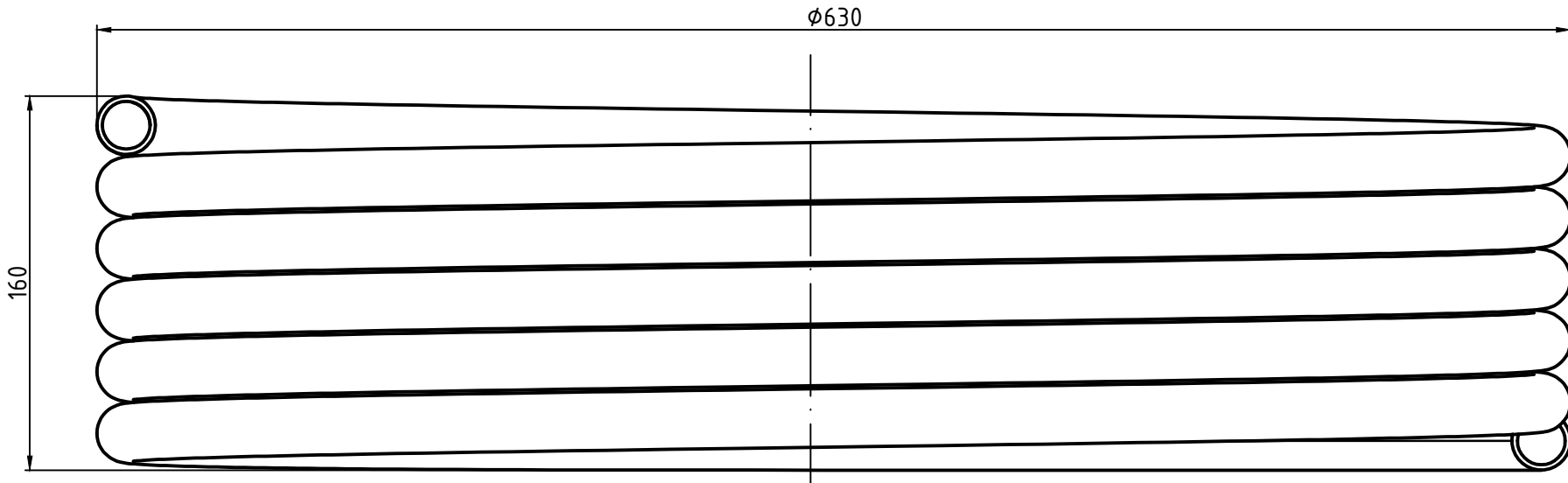
Querschnitt M2:1
