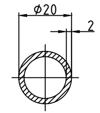
Querschnitt M2:1
