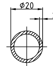
Querschnitt M2:1
